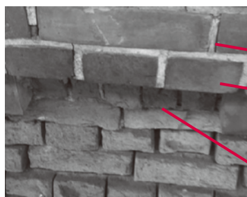
←写真3 二階腰壁部分 水切り部分 「焼き過ぎ」煉瓦 窯外部壁面の風化
